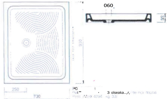
60794 PIATTO POLO 73x91 BIAN
