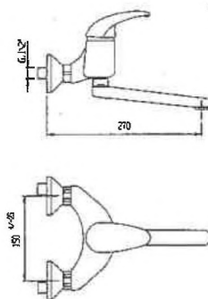
72726 MIX DOCCIA EST. BARI CRO MPB Art. 3430 P/C. 1
