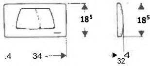
Placca di copertura con doppio tasto di comando
