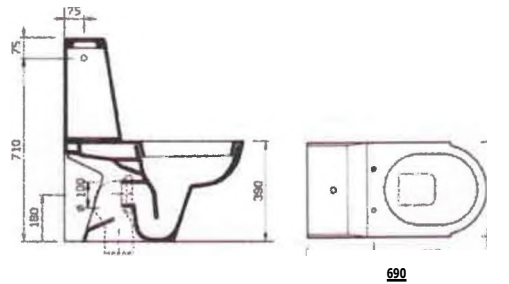
MONOBLOCCO ZAGARA - CASSETTA ART. 3240 Vaso e cacciata Scatto a potete. L'installazione a prunzie a+ effettua can reposita curve 1~3 ART. 9303 Cmgetto cori coperCha. POSO vaso Kg. 27 crea - cassetta Kg 12 crea
