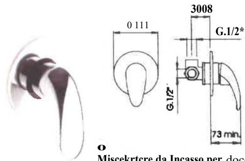
73838 MIX EST DOCCIA TALENTO CR SOL Art. 14258.002 P/C.1
