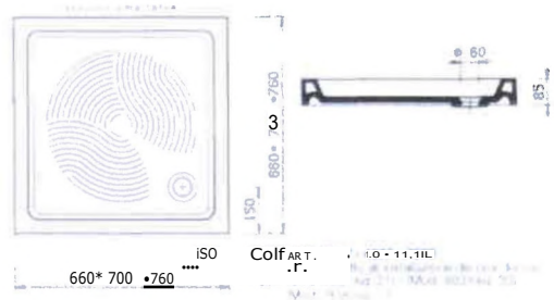
60790 PIATTO GOLF 66 BIAN
