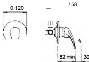
73895 MIX INC DOCCIA SMART CR sa Art. 02262R001-C P/C.1
