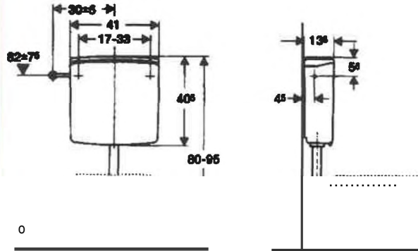
79082 CASSET EST 6/9 LT CHAMPAGN GEB Art. 140301.39 P/C.1
