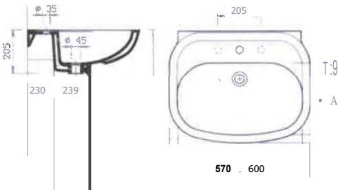
LAVABO RIO ART. 2200/ S00 COLA COLOW 2210 Cambilezione " " muro con bulloni 28 Cod. 60113) Peso: lavabo
