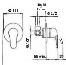
73864 MIX INCASSO DOCC PRIMA BIA. SOL Art. 13268-001NE
