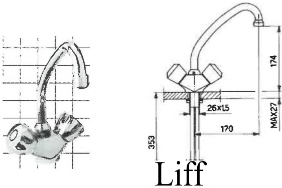
71204 GRUPPO LAVELLO MONOFORO T RAP Art. 8050700000 P/C.1
