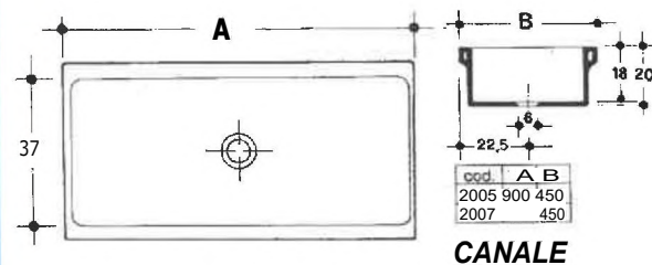
60840 LAVATOIO CANALE 90 BIAN GALArt. 2005
