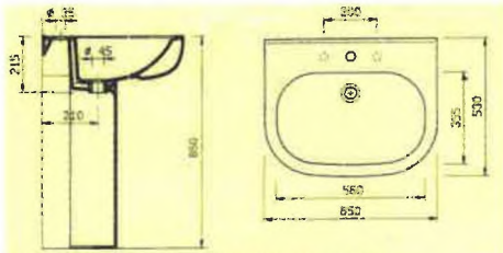
LAVABO ALPINA ART. 2600 CON COLONNA ART. 2210 Combinazione lavabo con colonna. Il lavabo viene fissato al muro con 000 bulloni. Peso: lavabo kg. 20 circa - colonna kg. 9 circa
