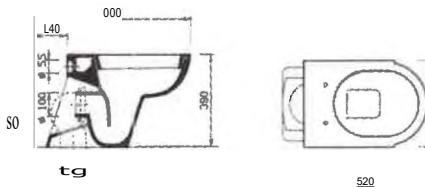
VASO ZAGARA ART. 3221 Valsa a cacciata. Scarico e penale lristatazione e ~mento ai effettua con apposita curva tecnica ART. 9303 n seciAa 8 fccr, to orettamente data Cerarrizza Oelcrite. P003: Kg. 24 circa
