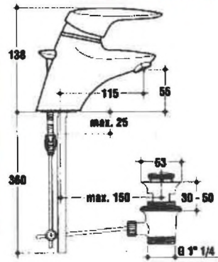
73275 CERA MIX 2000 GR LAVABO CR IDE Art. A5011M P/C.
