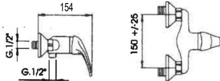
73896 MIX EST DOCCIA SMART CR sa Art. 02262A002-C P/C.1
