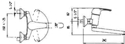
Miscelatore a parete per lavello, bocca lusso girevole.
