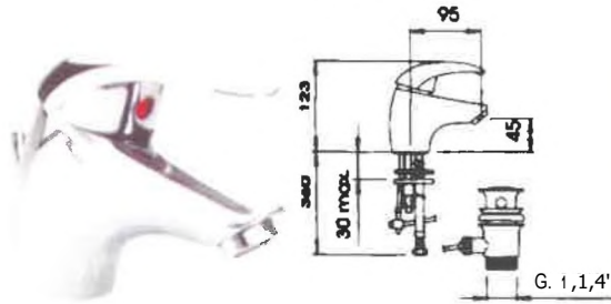
73834 MIX LAVABO TALENTO CR SOL Art. 14358-001 P/C.1
