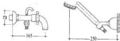
73218 TALENT GR VAS CROM IDE Art. N9054GY P/C.1
