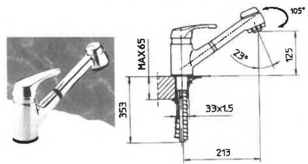
71139 MISC. LAV. DOCC/ESTR. MK3 RAP Art. 9222142000 P/C.1
