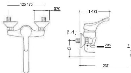
73214 CERAMIX GR LAVEL PAR IDE Art. A 2520 P/C.1
