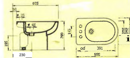
BIDET ALPINA ART. 2632-2634 li Mod. 2632 a tre fon [previste] con erogazione dell'acqua a zarin 3 p ti 7.0 L.V. li Mod. 26344 monotono con erogazione dell'acqua dei rubinetto. Peso. 59,17 crea.
