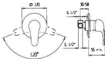
Miscelatore da incasso per doccia. Con cartuccia normale Globo.
