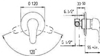
Miscelatore da incasso per doccia. Con bilanciatore di pressione. Con cartuccia normale Globo.
