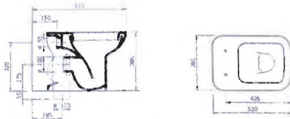
VASO RIO ART. 2221 Vaso a cacciato scarico a pessa Leatallabona a pavinienio 90190100001'ammala or,* rampa ARI 9303 h sedAs pot:forma ~mamma dea* Ganace. 3n10mae Paao k4 20 19019
