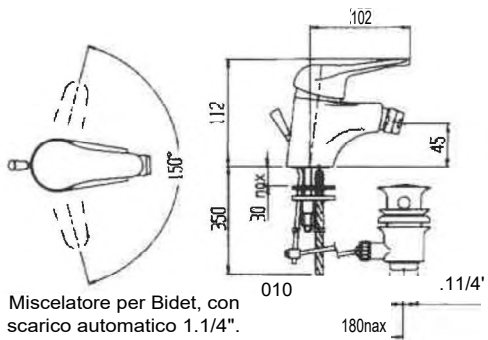
73503 MIX BIDET PUNTA CR SOL Art. 11476-001 P/C.1
