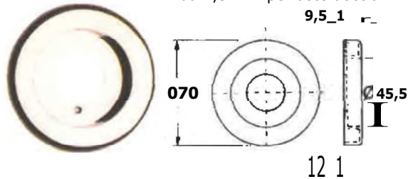
74719 DISTANZIATORE x ASTA GRO Art. 45459 P/C. 1
