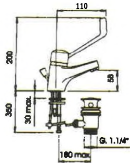
Miscelatore per lavabo tipo Punta con scarico automatico 1.1/d" con 1~ lunga
