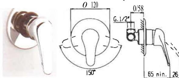
Miscelatore da incasso per doC0a
