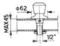
71203 RUBINETTO LAVABO 1/2 T RAP Art. 8030000000 PIC.1
