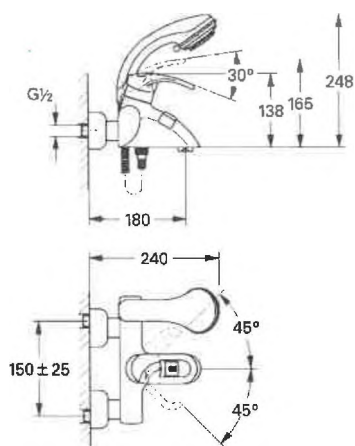
70772 CHIARA MIX VASCA CROMO/ORO GRO Art. 33419 IG P/C.1
