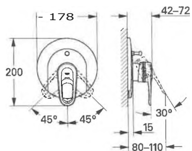
70680 EUROPLUS DUE ROSONE C/D.CR GRO Art. 19536 P/C.1
