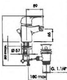
73862 MIX BIDET C/S PRIMA BIA SOL Art. 13468-001NE/P/C.1
