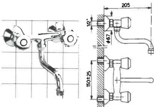
71214 GRUPPO LAVELLO A MURO T RAP Art. 6610700000 P/C.1
