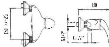
73838 MIX EST DOCCIA TALENTO CR SOL Art. 14258.002 P/C.1
