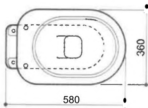
62504 VASO SINTESI BIAN CSM Art. 76200
