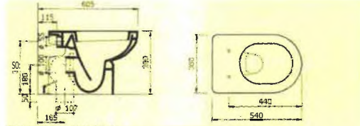
VASO ALPINA ART. 2021 Vaso a cacciata Scarico e parete. L'erstanarare a pavimento si *stette con apposita curva tecnica Art. 9303.11aedile può essere 1o251e dincttamente clan a Cerermca Date: nue Peso: 19, 20 area.
