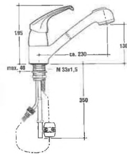
73204 MIX LIVELLO DOC/ESTR IDE Art. A2715AA A/C.1
