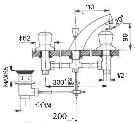
71201 BATTERIA LAV C/SALT. 1 T RAP Art. 8000000000 P/C.1
