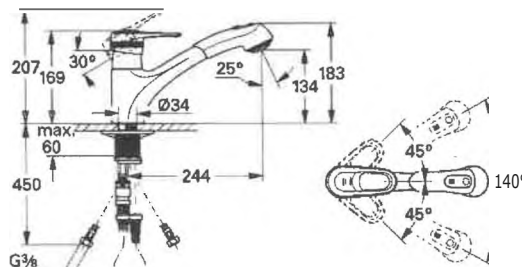
70677 EUROPLUS DUE LAVELLO C/DOC C GRO Art. 33933 P/C.1
