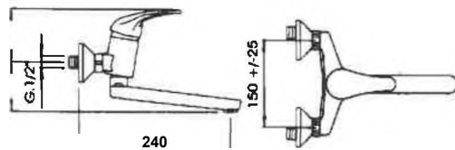
73897 MIX LAVELLO PAR SMART CR sol Art. 02562R002-CP/C.1
