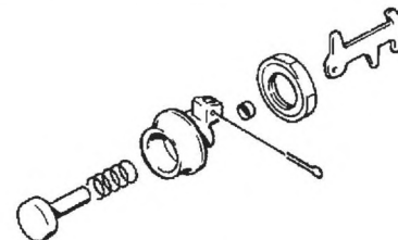
78528 GRUPPO PULSANTE TONDO FAI Art 3770015 P/C.1
