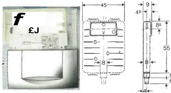
79011 CASSETTA INCAS. L 10 C/TUB GEB Art. 110700.00 P/C.1
