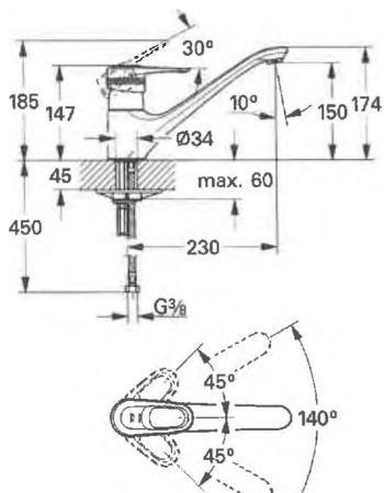
70676 EUROPLUS DUE LAVELLO CR GRO Art. 33930 P/C.1
