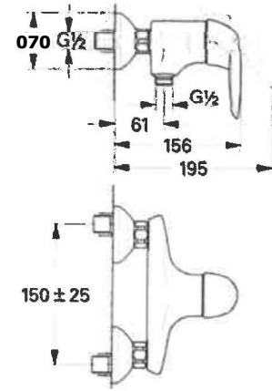
70618 EURODISC MIX EST DOCCIA GRO M. 33570
