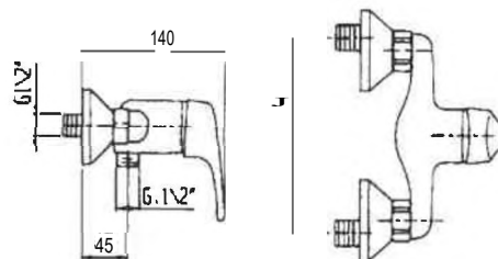
Miscelatore Esterno per Doccia, senza flessibile e doccetta, uscita inferiore da 1/2\".
